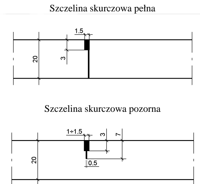
Rys. 1.1. Przykłady konstrukcji szczelin w podbudowie z betonu cementowego (wymiary w cm)
