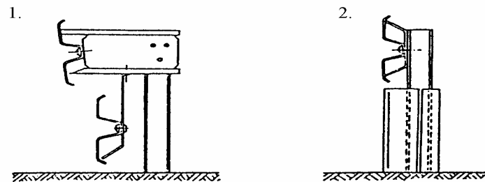
Załącznik 11.6. Sposoby lokalizowania barier w przekroju poprzecznym drogi, wg [32]
