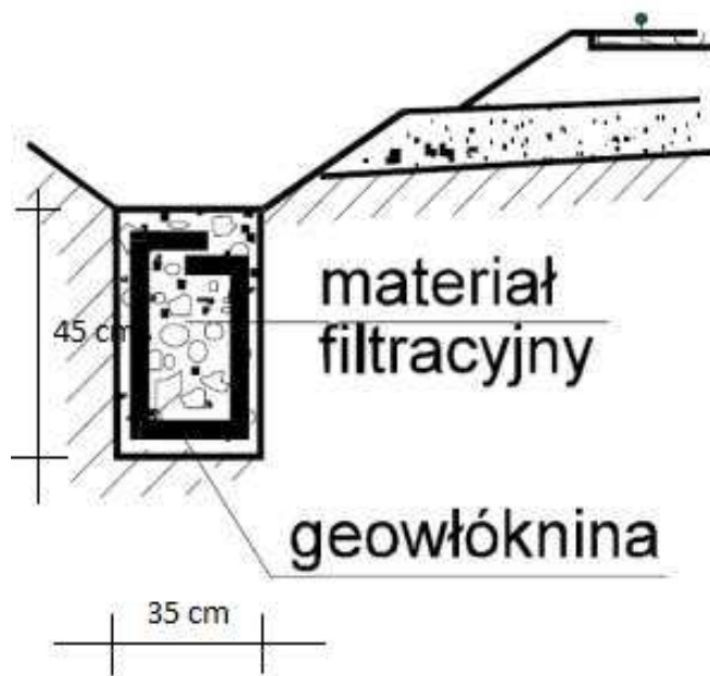
Schemat drenu francuskiego
