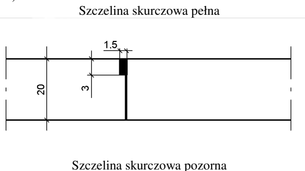
Rys. 1.1. Przykłady konstrukcji szczelin w podbudowie z betonu cementowego (wymiar w cm)
