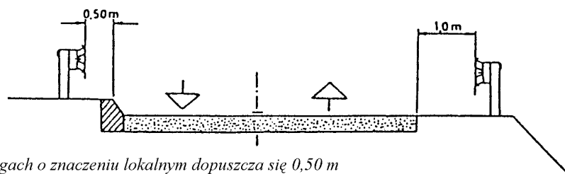
Załącznik 11.7. Zasady stosowania barier ochronnych stalowych na odcinkach dróg (wyciąg z WSDBO [32])
