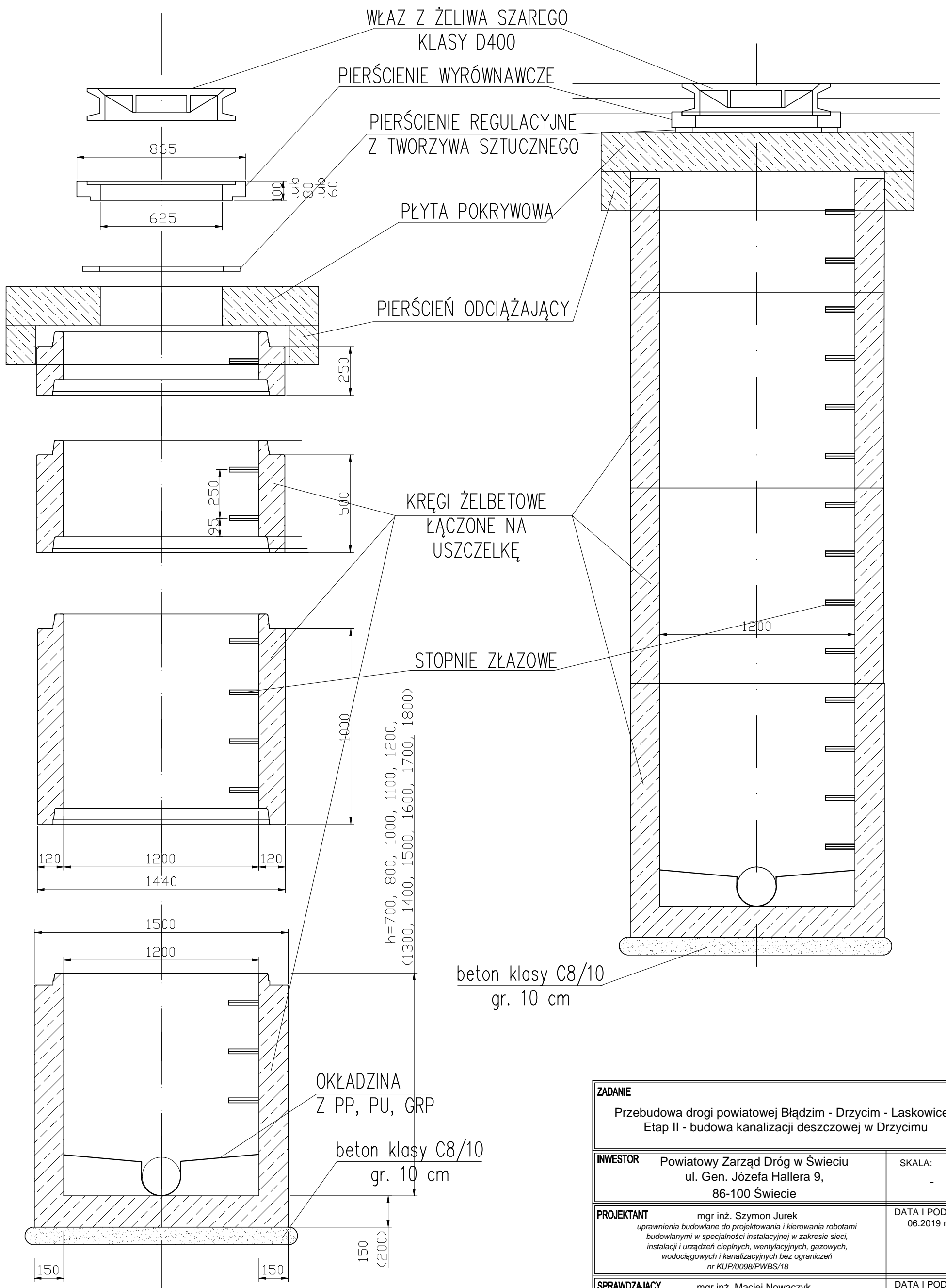
DENNICA NA PROJEKTOWANYM KANALE DESZCZOWYM Z FABRYCZNIE OSADZONYMI PRZEJŚCIAMI SZCZELNYMI
