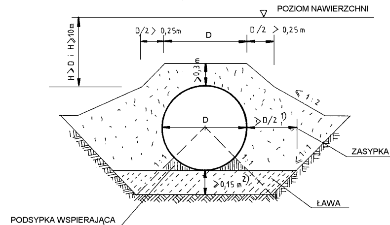
Rys. 8. Zasyпка nad przeputem jednorurowym
