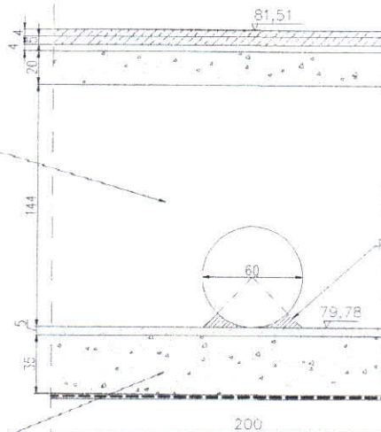
Przekrój A-A
