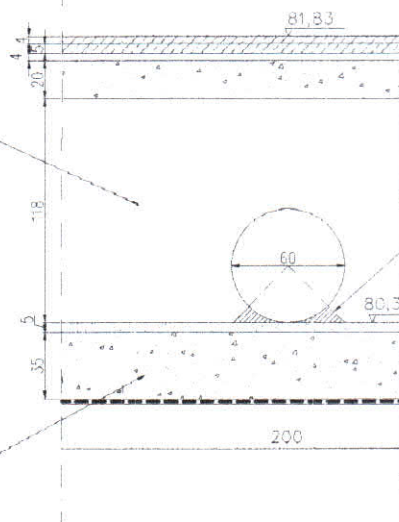
Przekrój A-A
