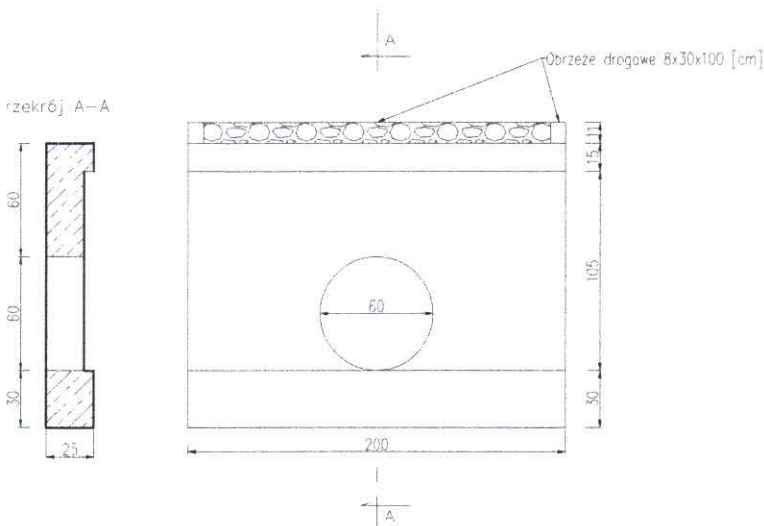
Widok projektowanego przepustu
