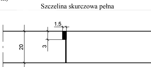
Rys. 1.1. Przykłady konstrukcji szczelin w podbudowie z betonu cementowego (wymiarzy w cm)
